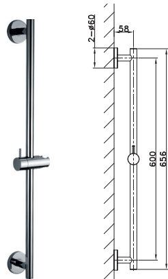
Barre de douche
